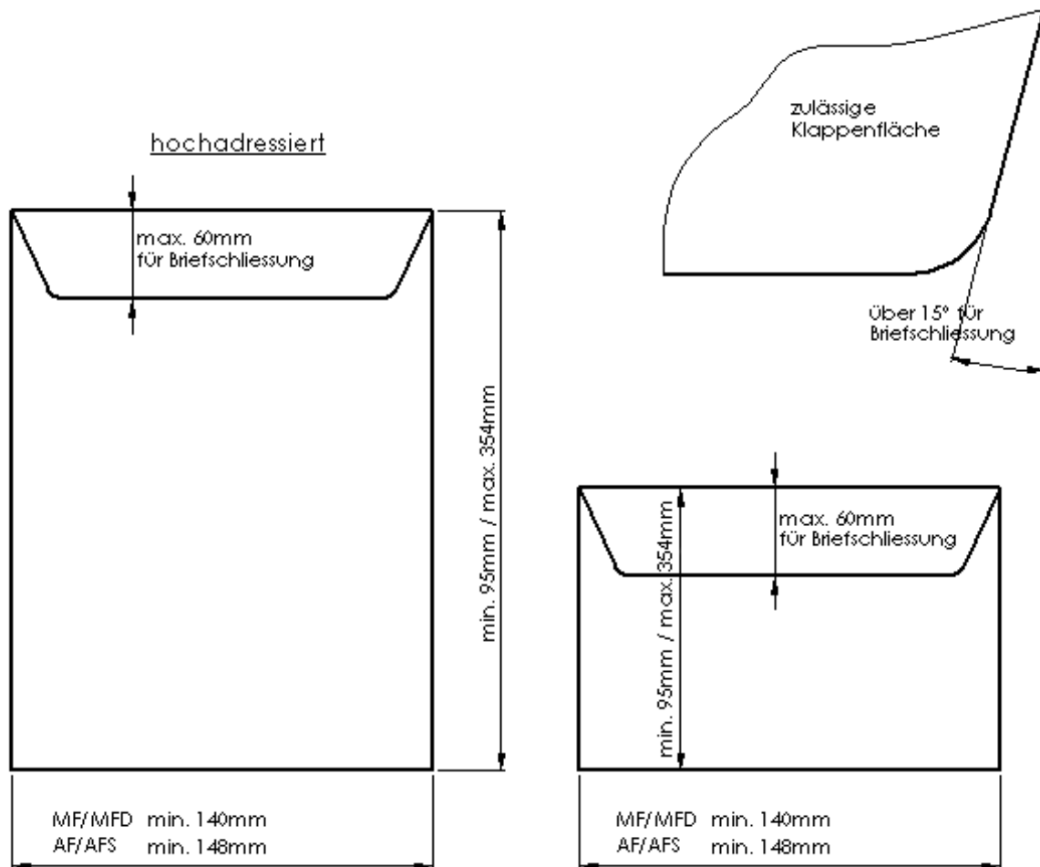
Obrázek: Specifikace chlopně obálky pro zalepovač dopisů / maximální a minimální specifikace obálky
